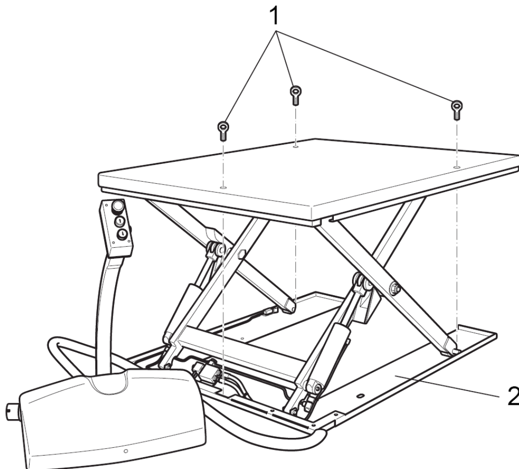
Rys. 6: Punkty mocowania na stole podnośnym (ilustracja przykładowa)
