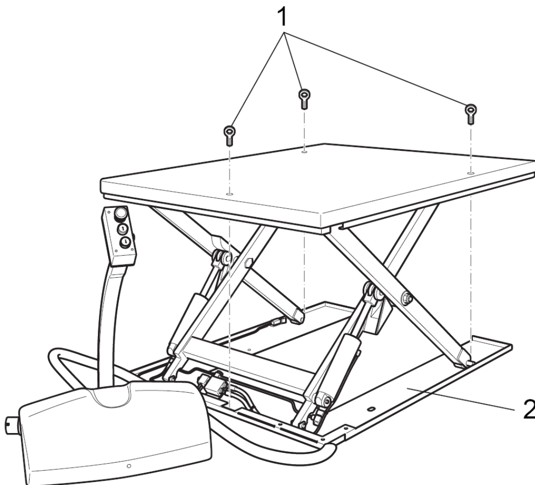
Ilust. 6: Puntos de enganche de la mesa elevadora (ilustración de ejemplo)
