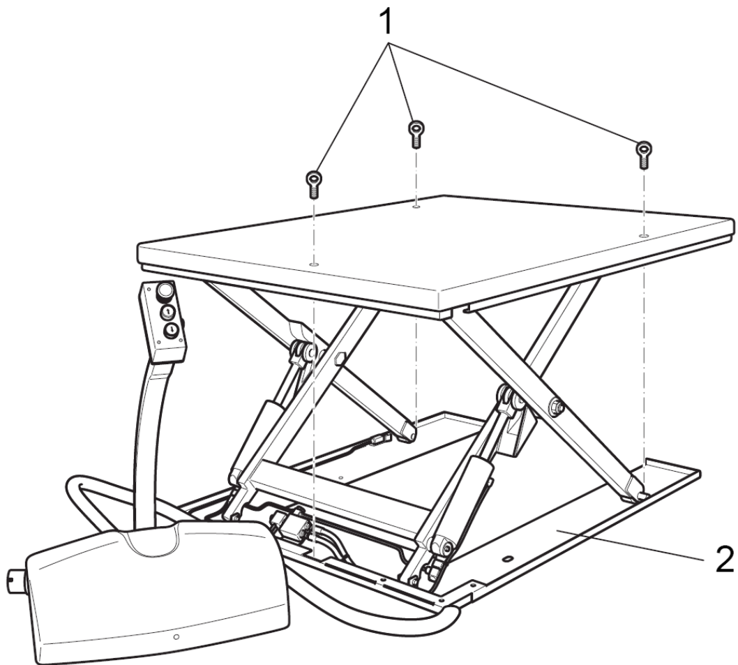
Fig. 6: Anhugningspunkter på løftebordet (eksempelvisning)
