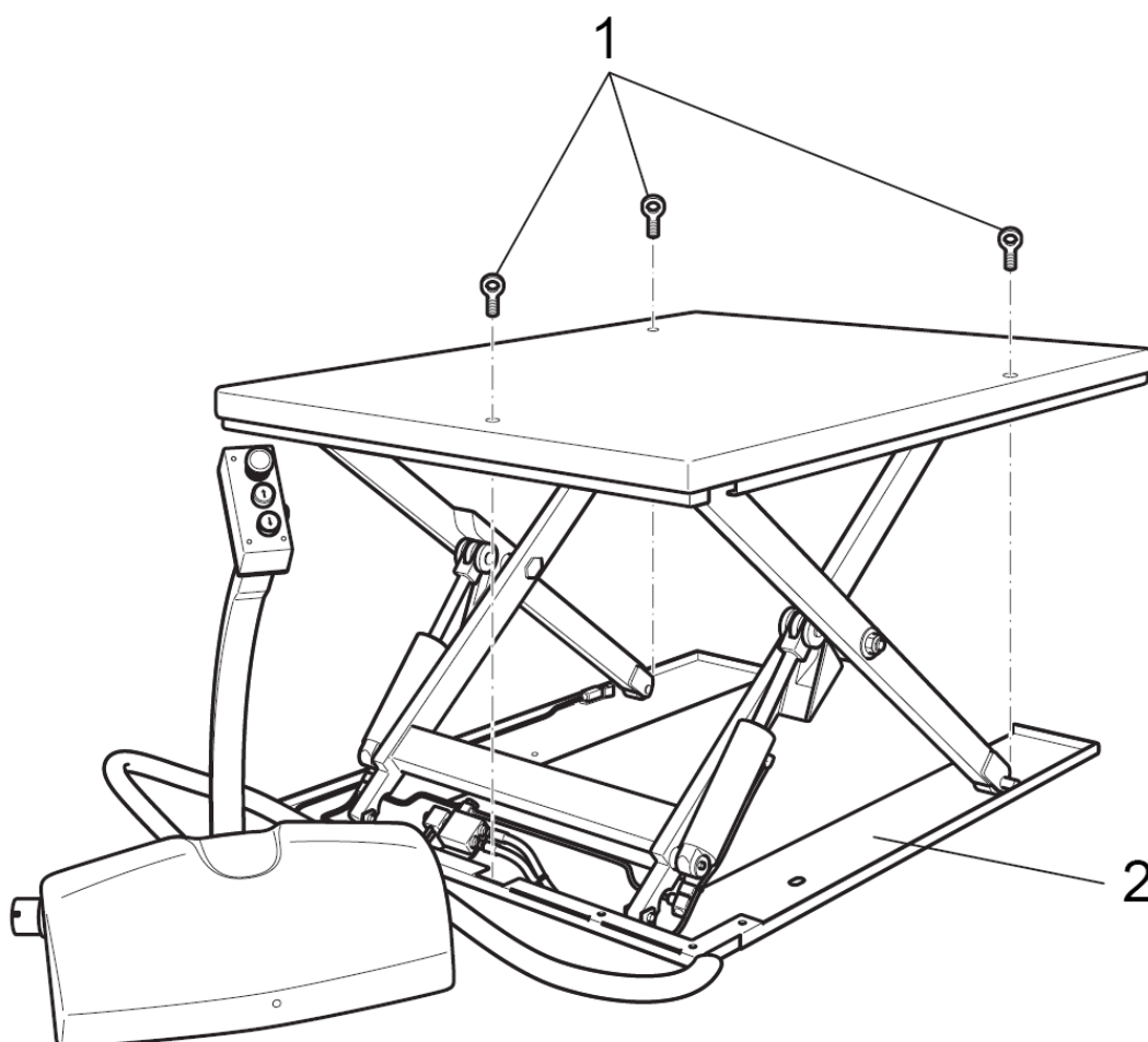
Ilust. 6: Pontos de fixação na mesa de elevação (representação exemplificativa)
