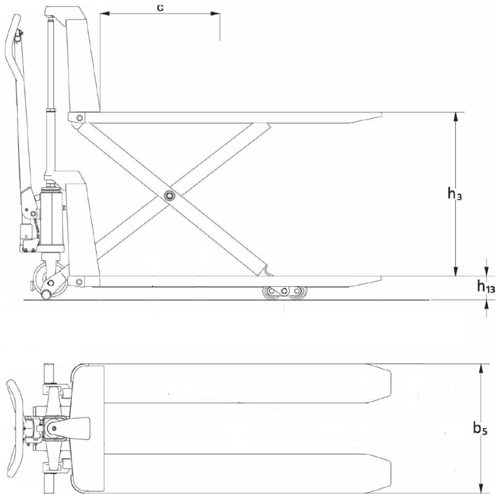
Abb. 3: Geräteabmessungen (Seitenansicht und Draufsicht, schematisch)
