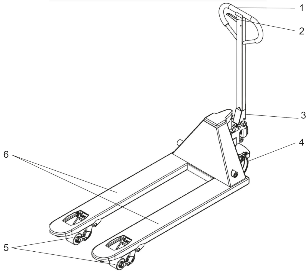
Abb. 1: Baugruppen- und Funktionsbeschreibung Flurförderzeug
