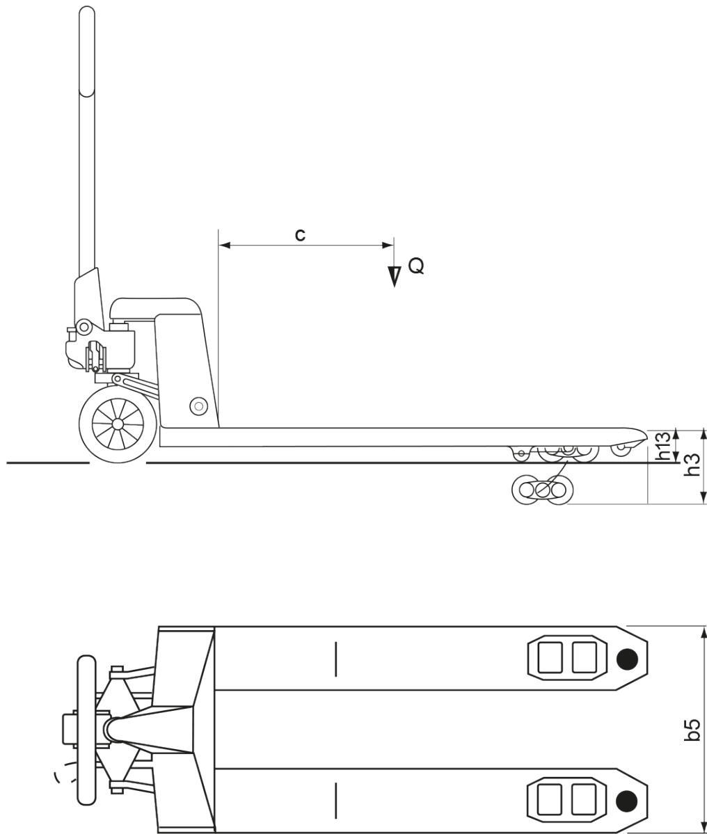
Abb. 4: Geräteabmessungen (schematisch)
