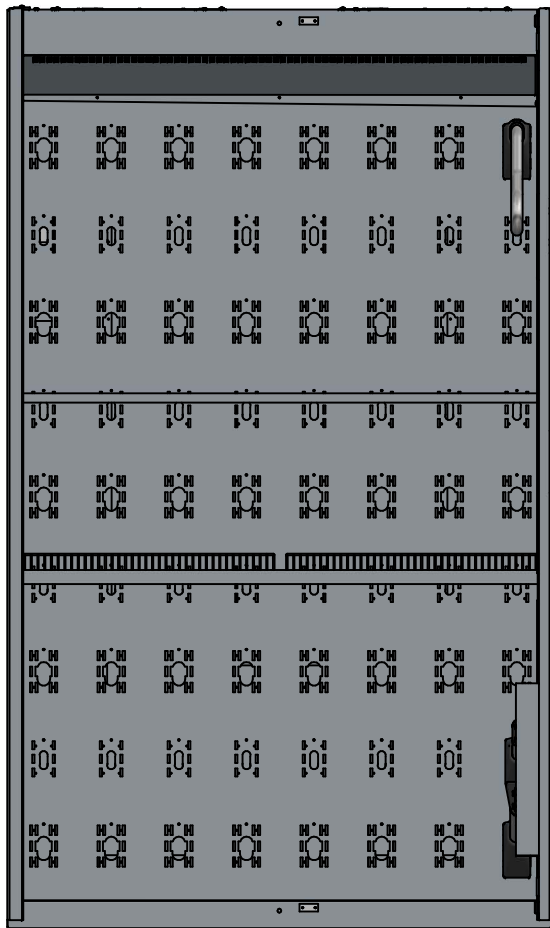
Vorderansicht
