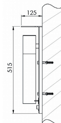
Modell 7061-01 Wandbefestigung
