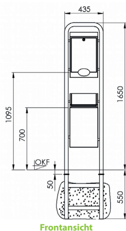
Frontansicht
