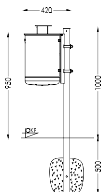
Pfostenbefestigung
