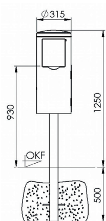
7077-00 Frontansicht zum Einbetonieren
