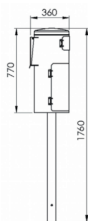
7077-00 Seitenansicht
