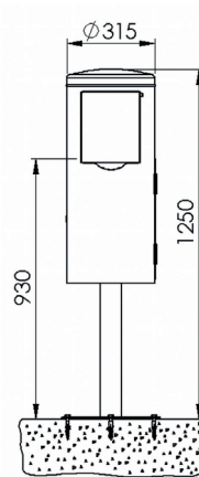
7077-01 Frontansicht zum Aufschrauben
