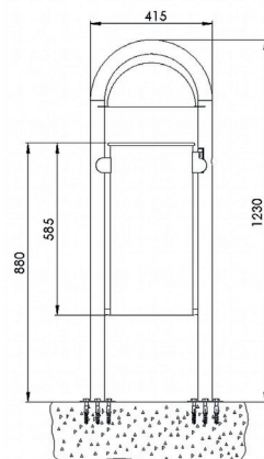
Frontansicht Ausführung zum Aufschrauben
