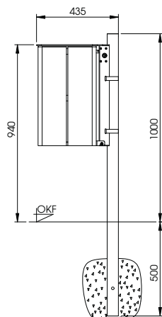
Pfostenbefestigung
