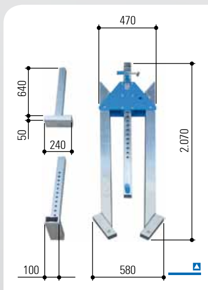
montante plegado
