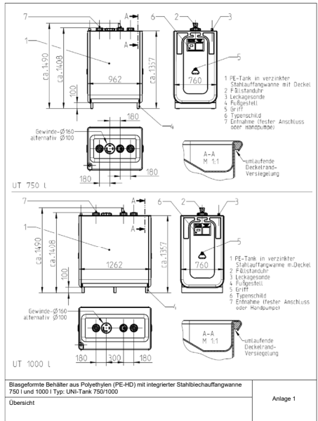
Blasgeformte Behälter aus Polyethylen (PE-HD) mit integrierter Stahlbeheizungsanlage 750 l und 1000 l Typ: UNI-Tank 750/1000 Übersicht
