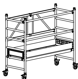
Gerüsttyp Größe 3 (Bestell-Nr. 53513)
