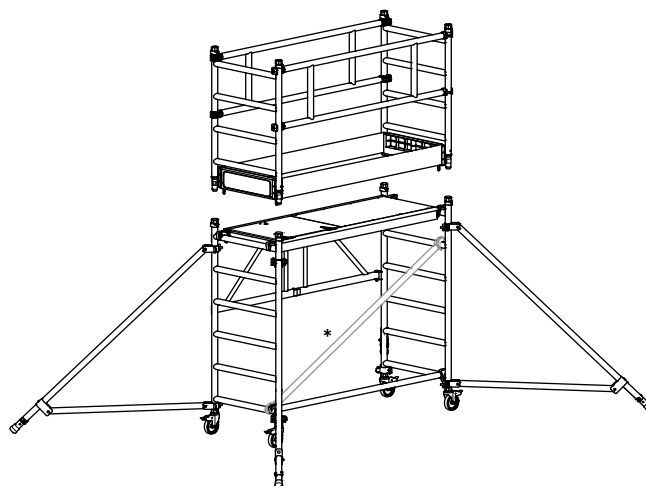
Gerüsttyp Größe 2 (Bestell-Nr. 53512)
