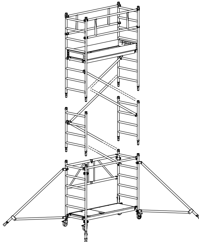
Gerüsttyp Größe 4 (Bestell-Nr. 53514)
