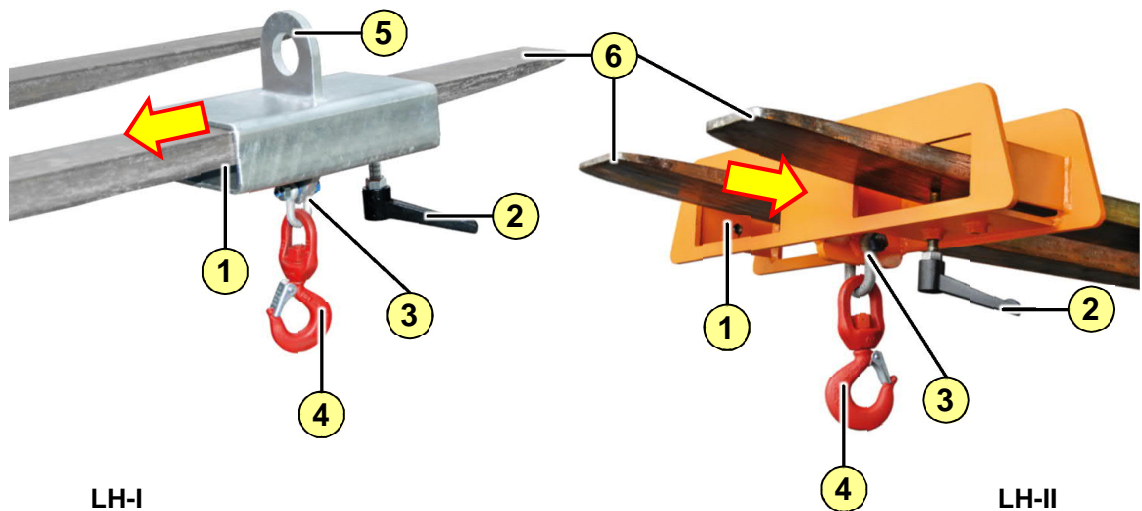
Abb. 5-1: Lasthaken nutzen
