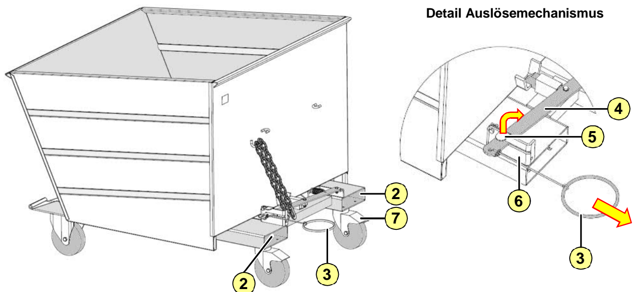
Abb. 5-1: Bedienen Kippbehälter
