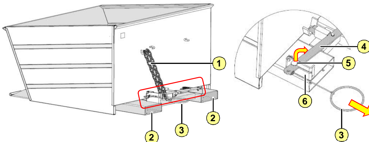
Abb. 3-1: Baugruppen Kippbehälter VD
