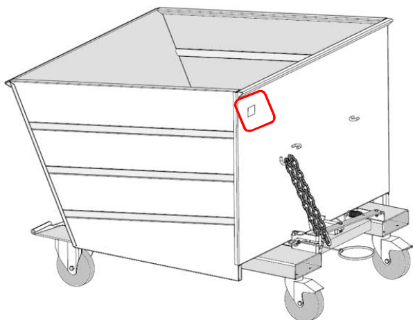
Abb. 2-2: Lage der Warnsymbole/Produktsicherheitslabel
