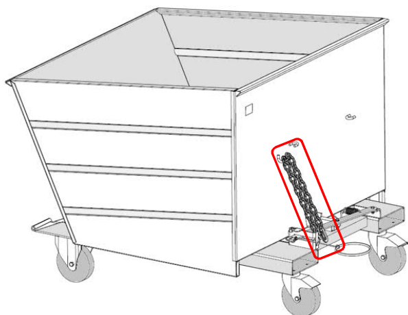
Abb. 2-1: Sicherheitskette am Behälter
