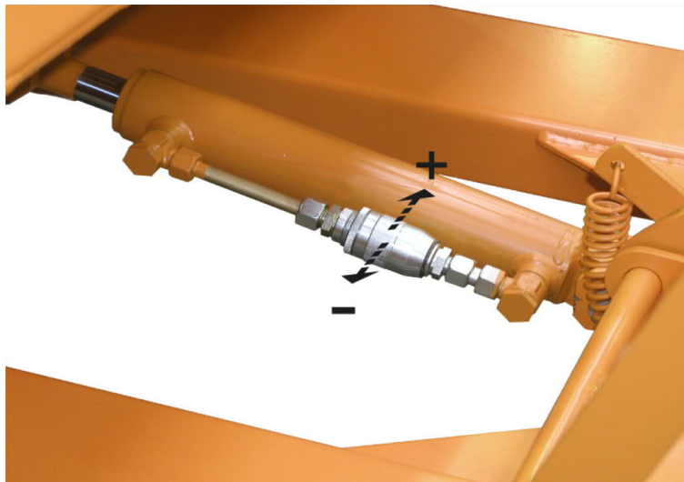
Abb. 5-4: Einstellen Kippgeschwindigkeit Kippbehälter
