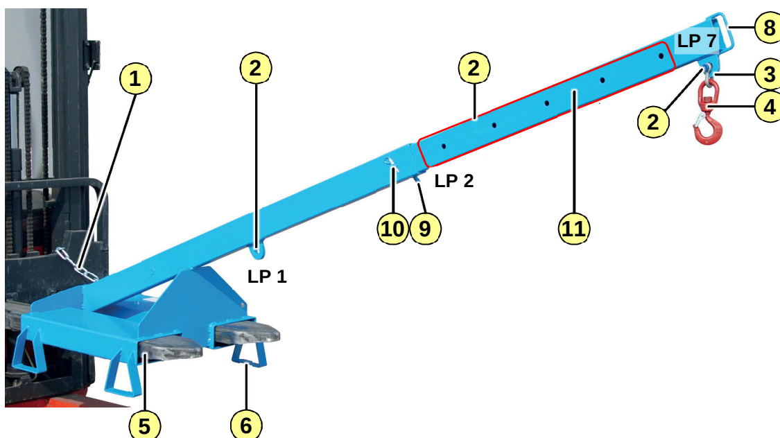
Fig. 5-3 : Sous-ensembles du Bras de chargement LAT 25-1.0
