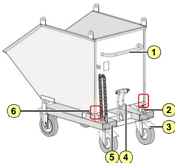
Fig. 5-1 : Commande de la Benne basculante / Benne basculante à copeaux
