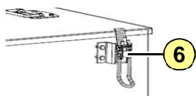
Fig. 5-3 : Fixer le couvercle
