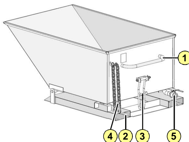
Fig. 3-2 : Sous-ensembles de la Benne basculante / Benne basculante à copeaux
