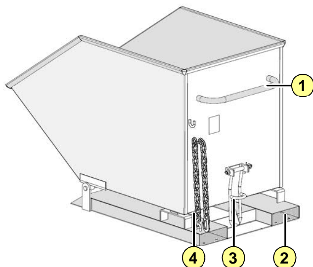
Fig. 3-1 : Sous-ensembles de la Benne basculante / Benne basculante à copeaux
