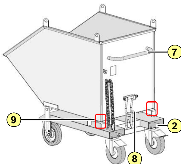
Fig. 5-4 : Commande de la Benne basculante / Benne basculante à copeaux
