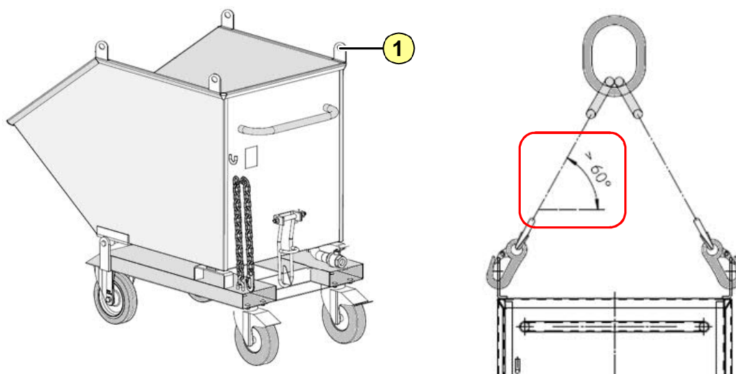
Fig. 5-1 : Transport avec la grue Benne basculante / Benne basculante à copeaux
