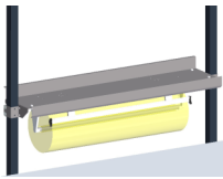
Standard Untertisch-Abroller mit Abreißschiene - glatt Rollenbreite: 500mm Best.- Nr.: 180150 Rollenbreite: 750mm Best.-Nr.: 180170
