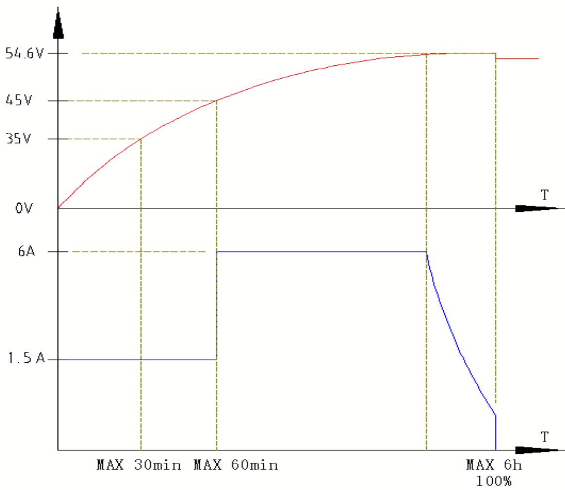
Ladekurve CBD 12W/LI und PTE 1.3
