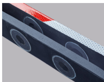
Je 4 Magnete auf der Innen- und Außenseite
