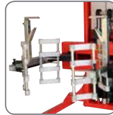
Flexible, speziell-entwickelte Greifarme lassen sich je nach dem Typ und dem Durchmesser des Fasses einstellen.
