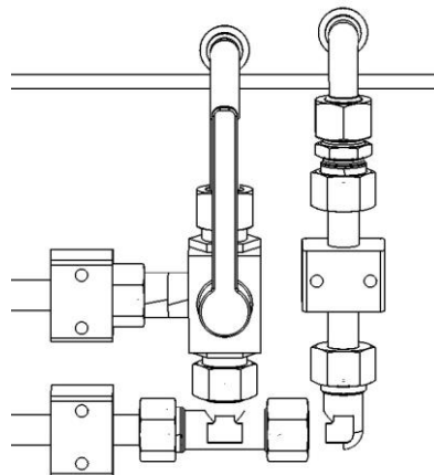
Abbildung 17 Hydraulik-Stellventil Seitenkehrbesen
