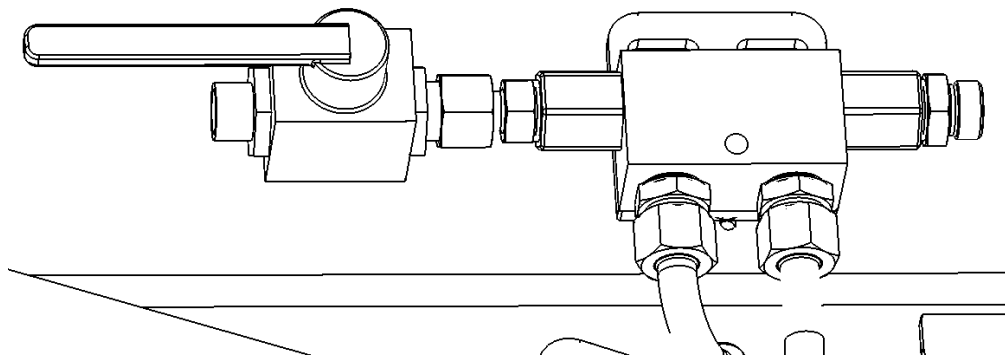
Abbildung 10 Hydraulik-Stellventil Freikehrmodus Schmutzsammelbehälter
