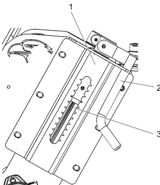
Abbildung 15 Höhenverstellung Kehrwalze
