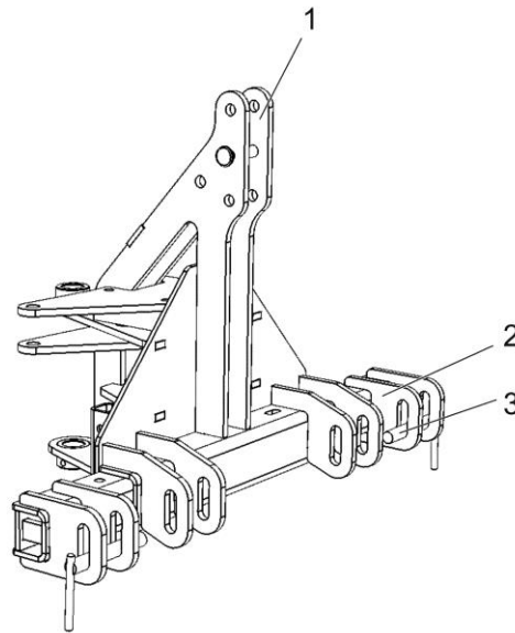
Abbildung 6 Dreipunktbock
