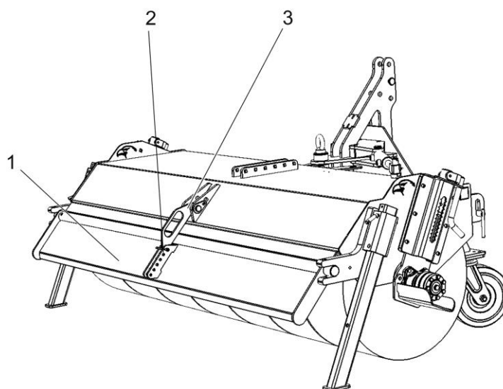
Abbildung 11 Verstellung Spritzschutzblech
