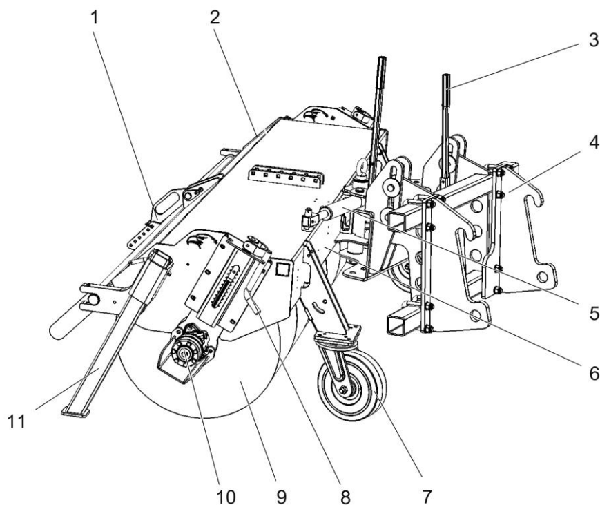
Abbildung 2 Kehmaschine K 600
