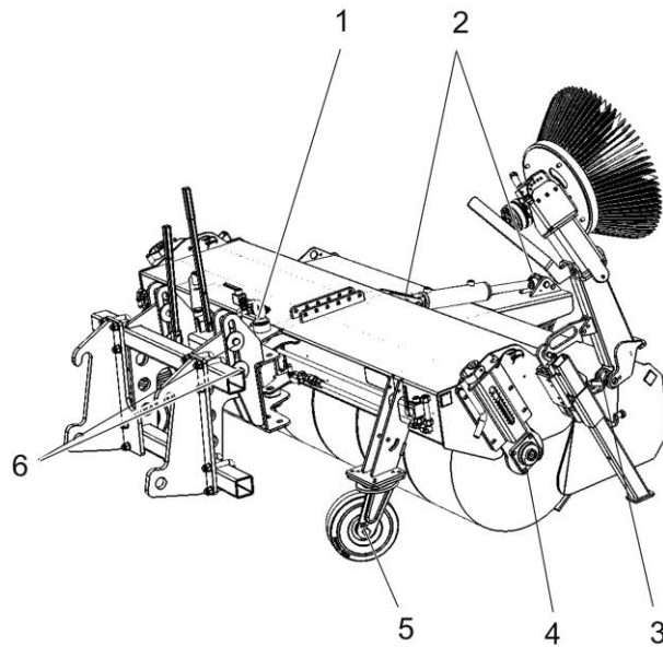
Abbildung 19 Schmierstellen
