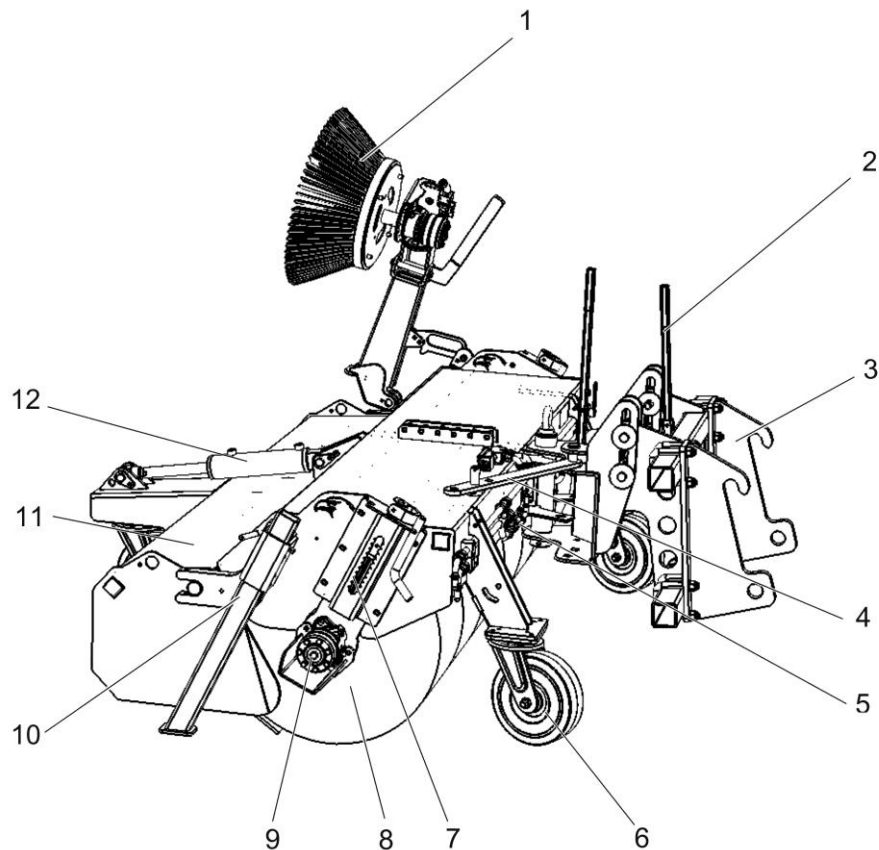
Abbildung 3 Kehmaschine K 600 Vollausstattung
