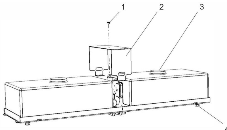
Abbildung 9 Wassertank 240 Liter
