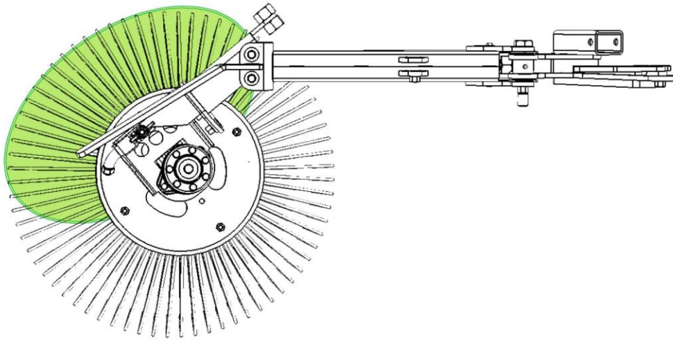
Abbildung 18 Eingriff Seitenkehrbesen
