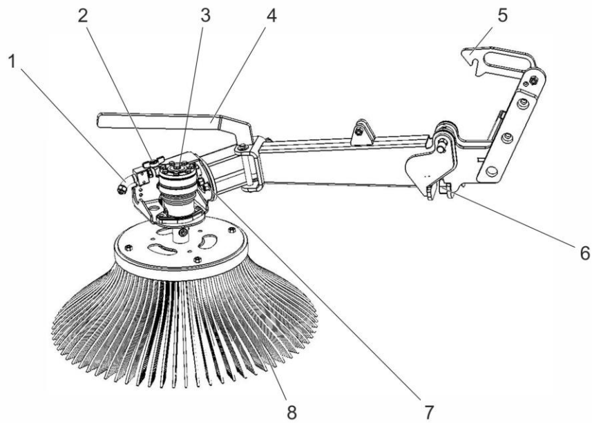
Abbildung 16 Verstellung und Arretierung Seitenkehrbesen
