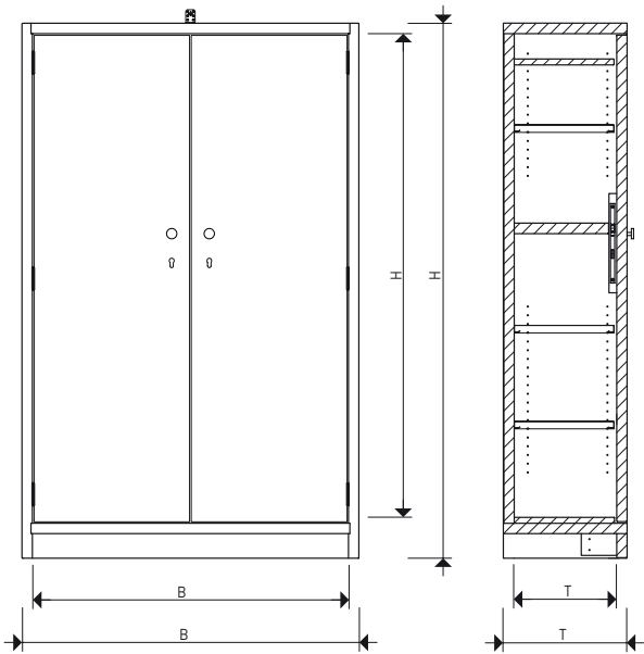
AS32-196-123 3 Einlegeböden | Shelves
