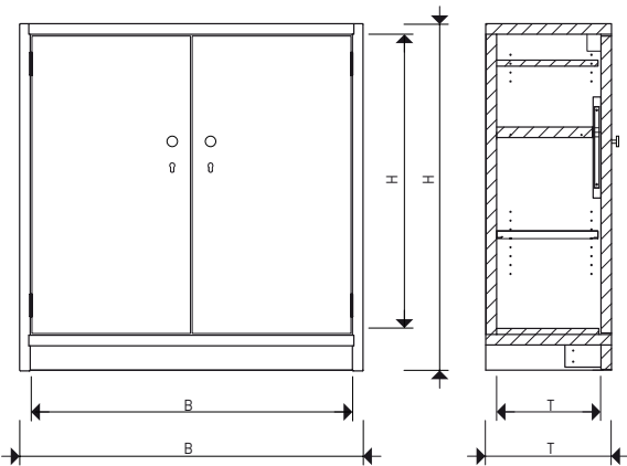
AS32-124-123 1 Einlegeboden | Shelf
