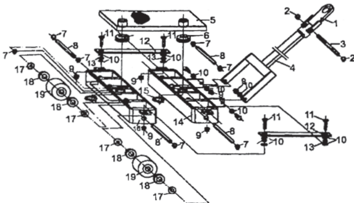
10. Eksplozivni crtež i popis dijelova za ST60
