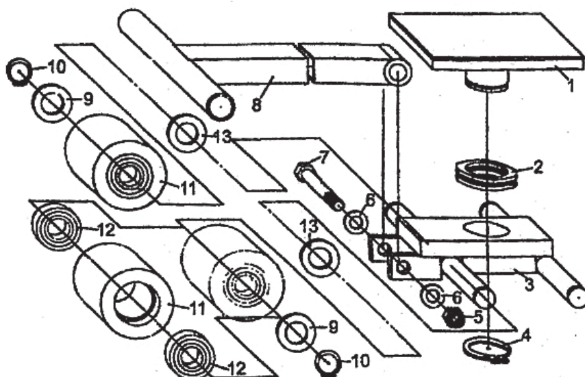
10. Eksplozivni crtež i popis dijelova za ST60
