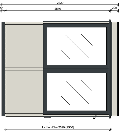
Vorderansicht
