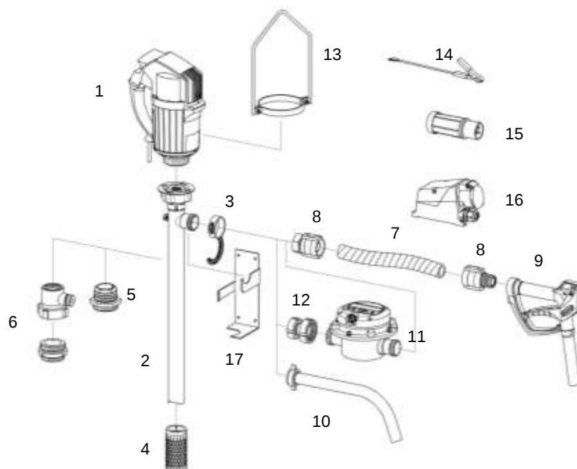
Fig. 1: Conception de la pompe antidéflagrante (avec composants)
