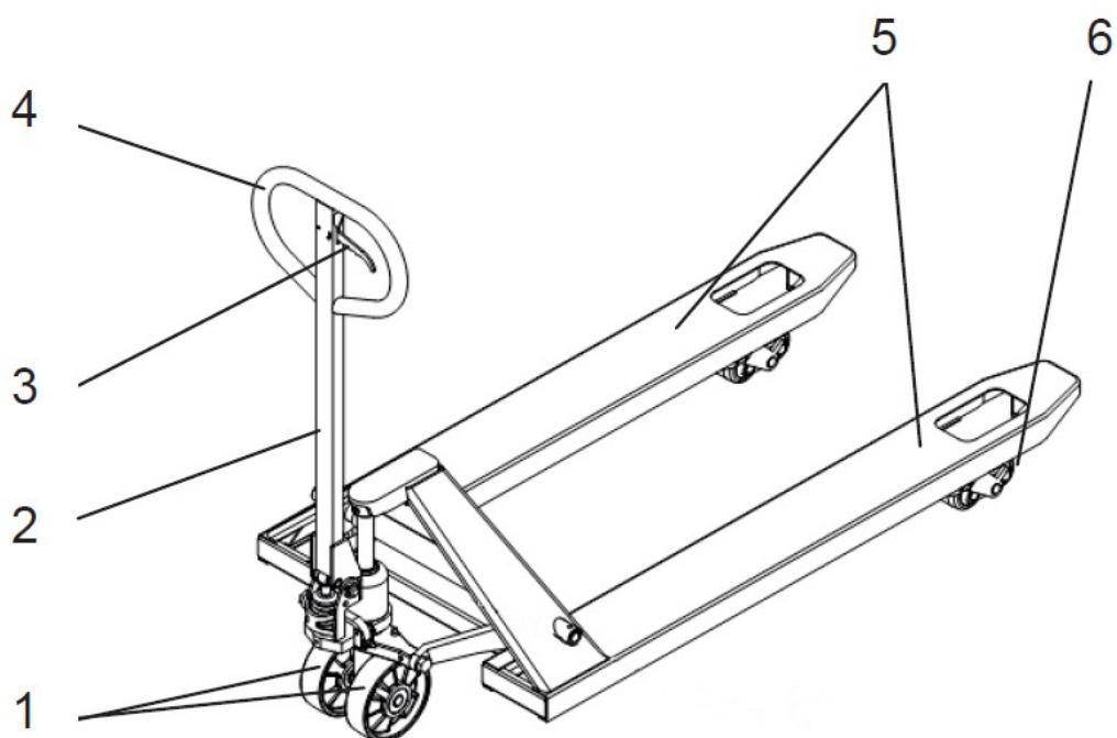
Obr. 1: Popis konštrukčných skupín a ich funkcie
