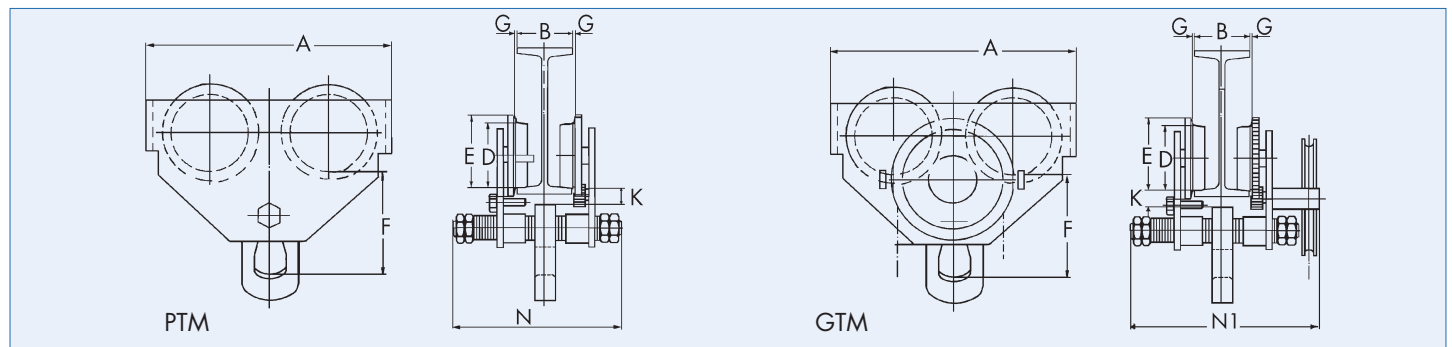
Haspelkettenlaufkatze GTM
