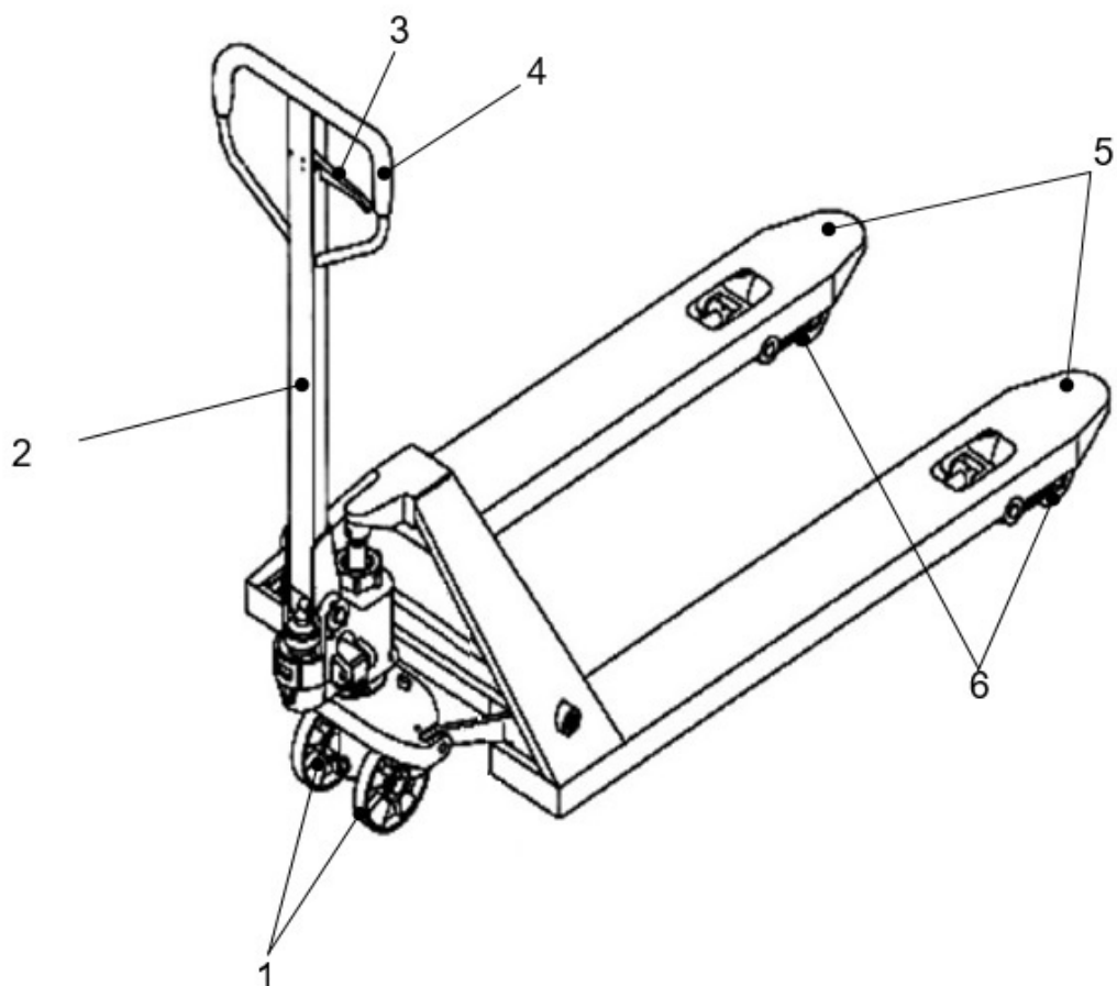
Rys. 1: Opis podzespołów i działania
