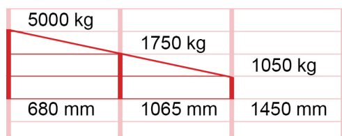
Traglastdiagramme für RLA-5 1500
