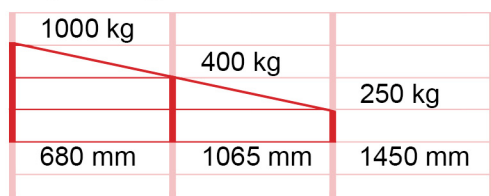
Traglastdiagramme für RLA-1 1500
