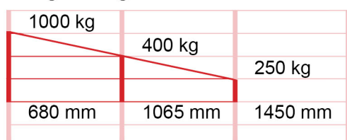
Draaglastdiagram RLA-1 1500
