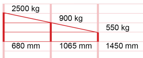
RLA-2,5 1500
