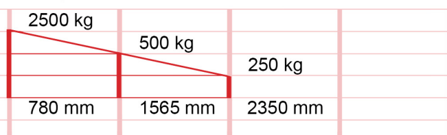
RLA-2,5 2400
