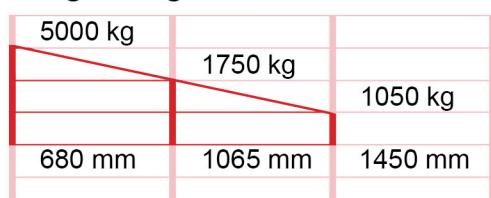
Draaglastdiagram RLA-5 1500
