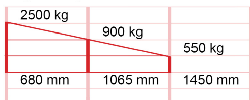
Traglastdiagramme für RLA-2,5 1500
