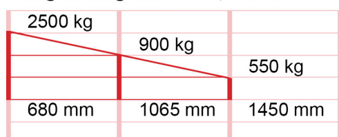
Draaglastdiagram RLA-2,5 1500
