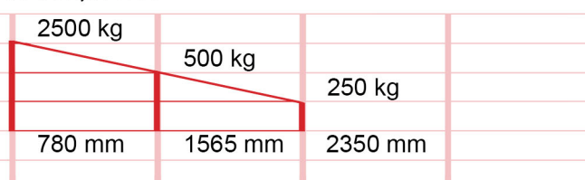
RLA-2,5 2400
