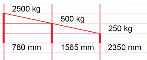
RLA-2,5 2400
