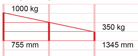
Draaglastdiagram RLH-1
