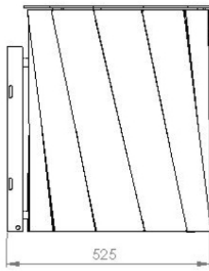
7007-20 Seitenansicht
